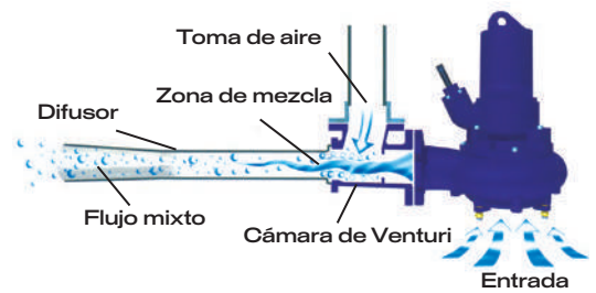
VENTURI-JET
